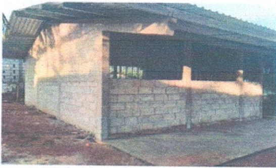
Foto1: Se observa elevada las paredes del módulo.
